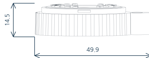
측면도 / SIDE VIEW
