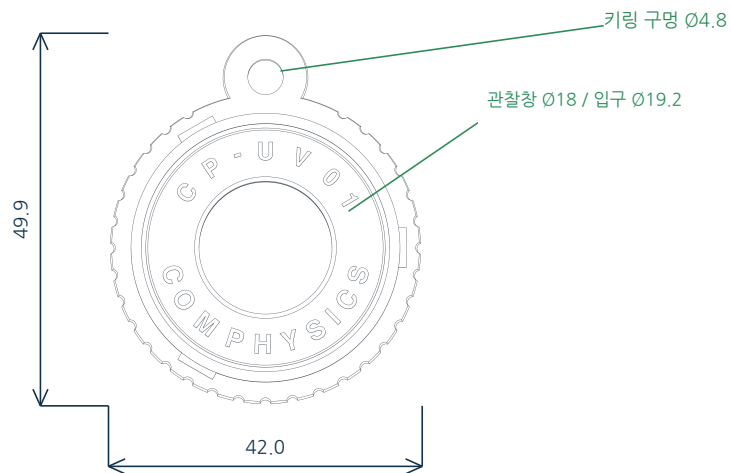
평면도 / TOP VIEW
